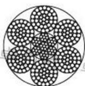
6*37+IWR
